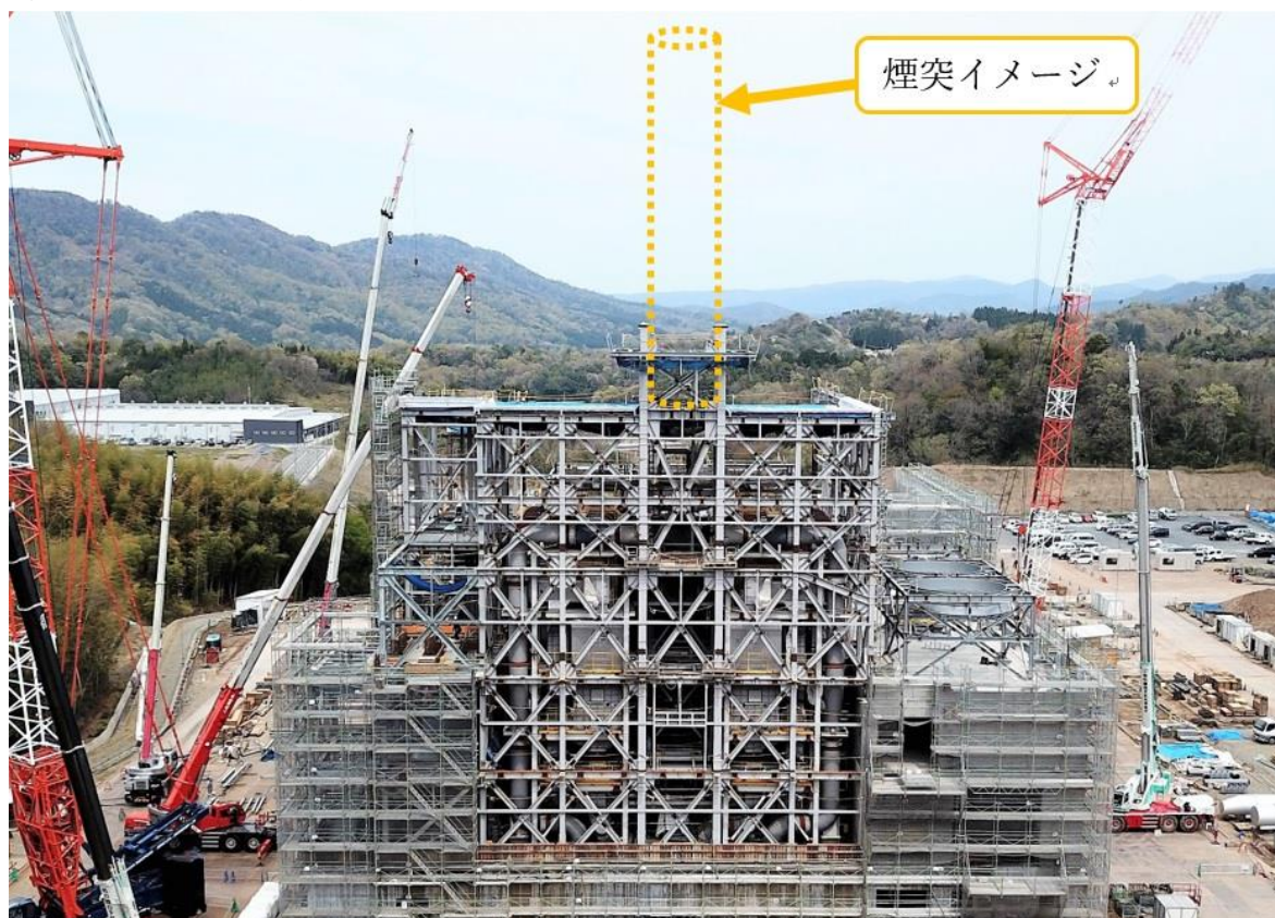
【排ガス処理エリア建築工事】
